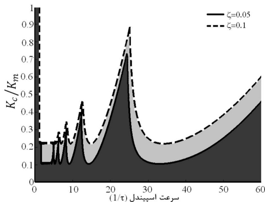
شکل 7 مقایسه ناحیه پایداری برای دو حالت \xi = 0.1 و \xi = 0.05 در \omega_n = 150
