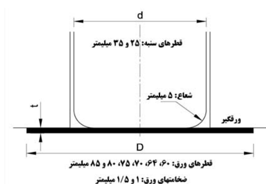
شکل ۳ طرحواره سنبه، ورق و ورقگیر در کشش عمیق هیدروفورمینگ
