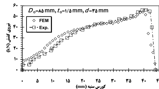
شکل ۶ مقایسه نمودارهای نیروی به‌دست آمده از آزمایش [۱۵] و
