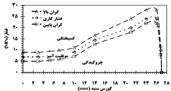
شکل ۱۲ نمودار کرن بالا و پایین فشار محفظه
