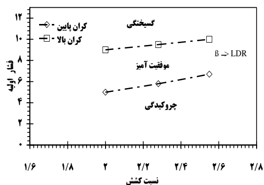
شکل ۱۳ نمودار کران پایین فشار اولیه برای نسبت‌های گوناگون گشش
