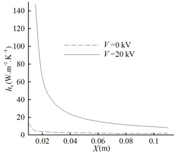
شکل 9 تغییرات ضریب انتقال حرارت موضعی در حالت روشن و خاموش محرک پلاسما (Re=250)
