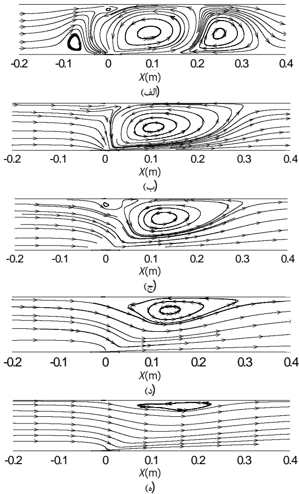
شکل 13 اثر عدد رینولدز بر روی تابع جریان در ولتاژ 20 کیلوولت Re=1000 (ه), Re=750 (د), Re=500 (ج), Re=250 (ب), Re=50 (الف)
