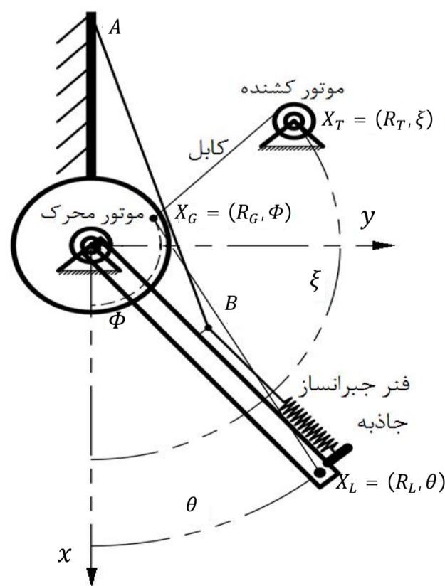
شکل 1 نمای شماتیک ربات توانبخشی
