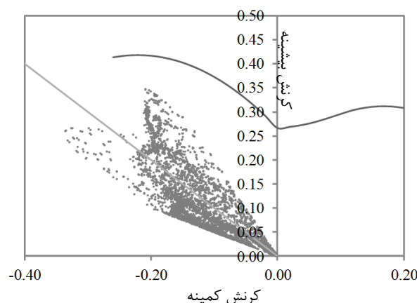
شکل ۹ نمودار حد شکل دهی قطعه صلیبی شکل
