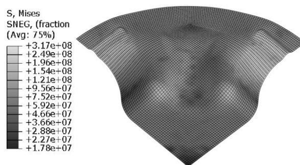
شکل ۱۰ کانتور قطعه صلیبی شکل
