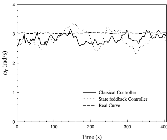
Fig. 12 Rotor angular speed curve in real and simulation state شکل 12 منحنی سرعت زاویه ای روتور در حالت واقعی و شبیه سازی شده
