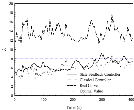
Fig. 11 Blade tip speed ratio curve in real and simulation state شکل 11 منحنی نسبت سرعت نوک پره در حالت واقعی و شبیه سازی شده
