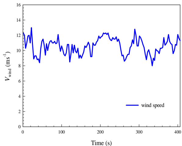
Fig. 10 Wind speed curve using in simulation شکل 10 منحنی سرعت باد مورد استفاده در شبیه سازی
