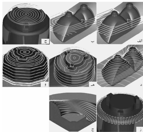
شکل 1 (الف) رستر (ب) آفست سه‌بعدی (ج) مارپیچ (د) پله‌ای بهینه‌شده و (ه) پله‌ای تفکیک‌شده (ز) شعاعی (ح) پرداخت سطح
