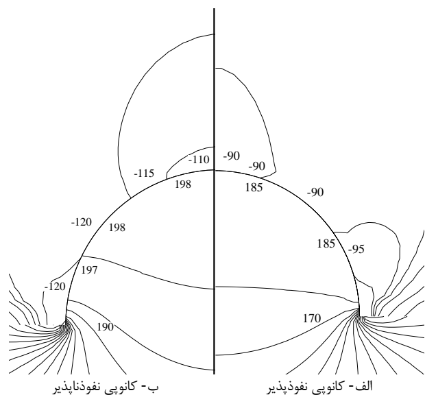
شکل 4 کانتور فشار دو سمت کانوپی
