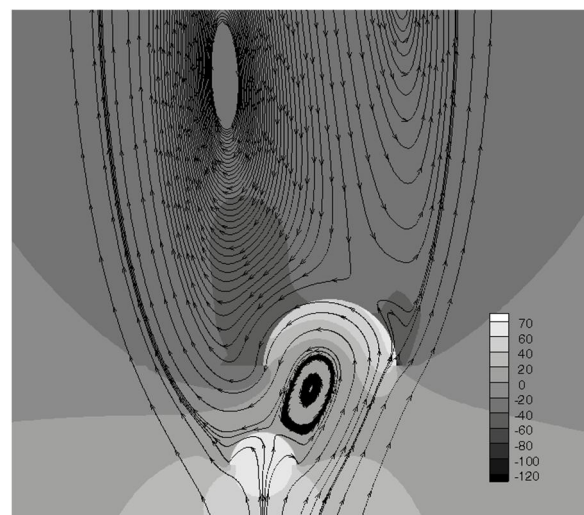
شکل 8 کانتور فشار و خطوط جریان در فاصله عمودی 1/5 و افقی یک برابر قطر
