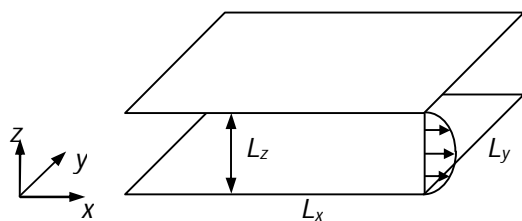
شکل 3 هندسه، دستگاه مختصات و ابعاد کانال
