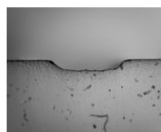
ب) در ولتاژ ۳۲V، عمق شیار ۹۴ \mu\text{m}
