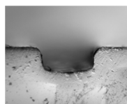
الف) در ولتاژ ۳۶V، عمق شیار ۲۷۵ \mu\text{m}
