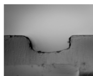
الف) در ولتاژ ۳۶V، عمق شیار ۲۵۴ \mu\text{m}
