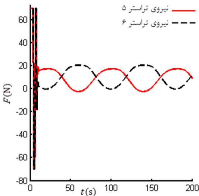
شکل 15 ورودی‌های کنترلی برای مسیر مارپیچ
