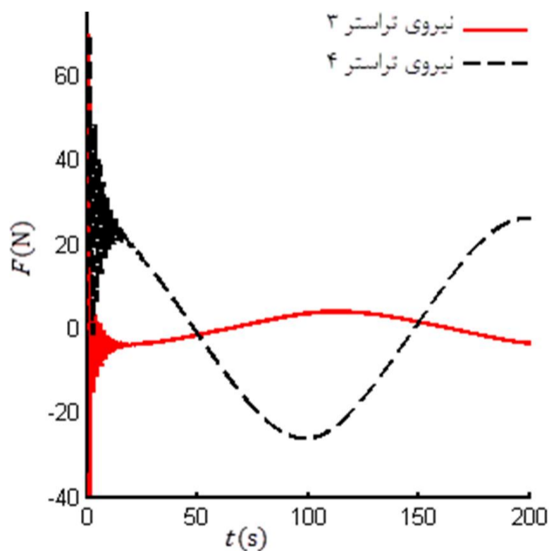
شکل 10 ورودی‌های کنترلی برای مسیر سینوسی در جهت‌های z و y
