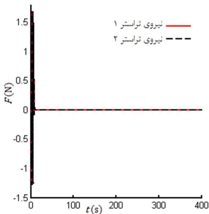
شکل 21 ورودی‌های کنترلی برای مسیر دایره
