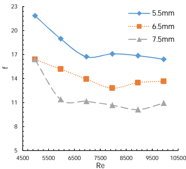
شکل 5 تغییرات ضریب اصطکاک برحسب عدد رینولدز
