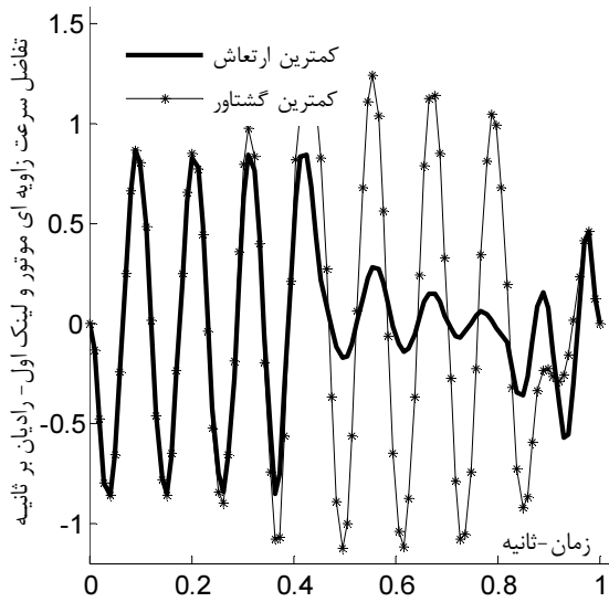
شکل ۱۰- الف اختلاف سرعت زاویه‌ای بین موتور و لینک اول
