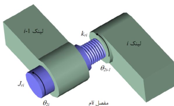
شکل ۱ شکل شماتیک مدل مفصل انعطاف پذیر
