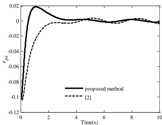
Fig. 3 error of x coordinate of the object in the straight line motion شکل 3 خطای محور x شی در مسیر مستقیم
