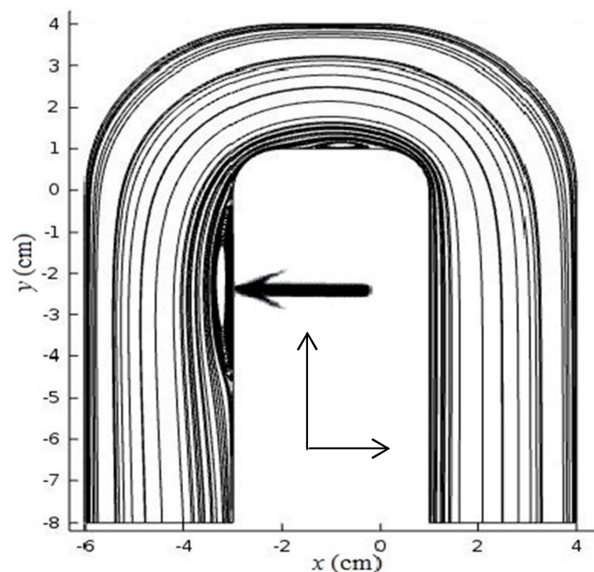
شکل 12 خطوط جریان در لوله و نقطه جدایش مورد نظر در رینولدز 6000
