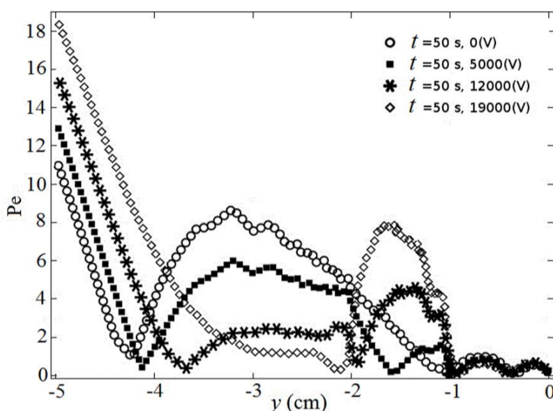
شکل 28 نمودار عدد پکلت در رینولدز 4500
