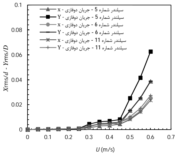
شکل 19 دامنه نوسان در جهت x و y برای حالت سه سیلندر متحرک (دسته سیلندر 19) - کسر حجمی 0/04 (3)
