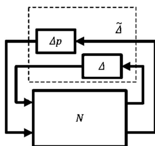
شکل 9 تبدیل بلوک دیاگرام به M-\Delta
