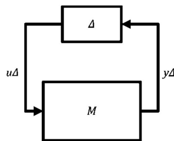
شکل 6 بلوک دیاگرام قالب استاندارد M-\Delta
