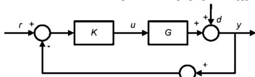
شکل 1 بلوک دیاگرام سیستم حلقه بسته
