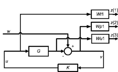
شکل 2 بلوک دیاگرام طراحی کنترلگر به روش حساسیت مخلوط
