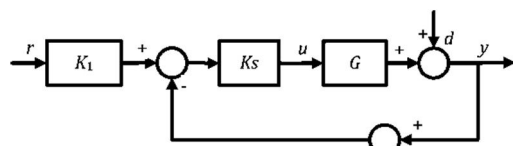
شکل 4 بلوک دیاگرام سیستم حلقه بسته دو درجه آزادی
