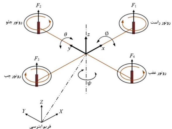
شکل 1 نمایی از دو دستگاه بدنی و اینرسی برای ربات پرنده چهارپره
