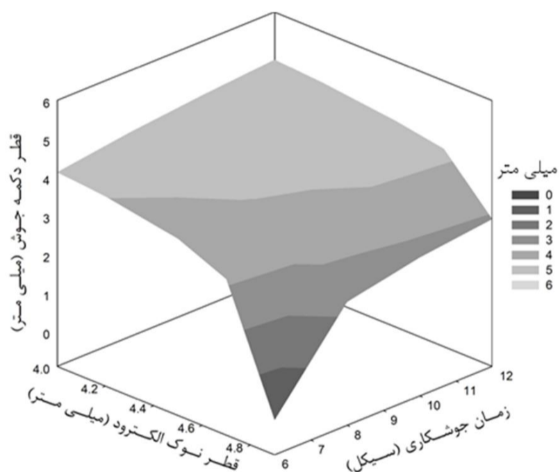
شکل 10 تأثیر متقابل زمان جوشکاری و قطر نوک الکتروود بر قطر دکمه جوش
