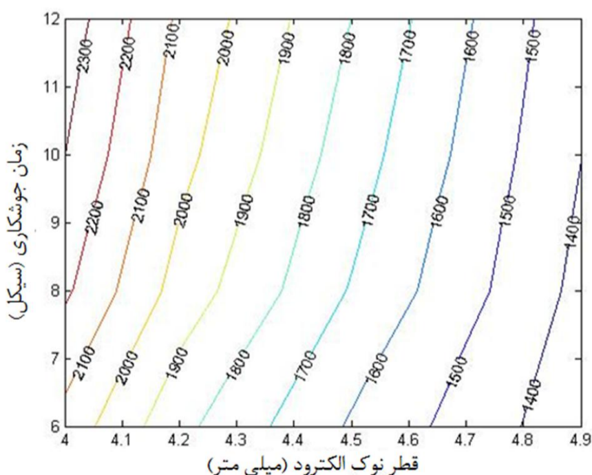
شکل 11 تأثیر جریان جوشکاری و قطر نوک الکتروود بر حداکثر دمایی دکمه جوش بر حسب درجه سانتی‌گراد
