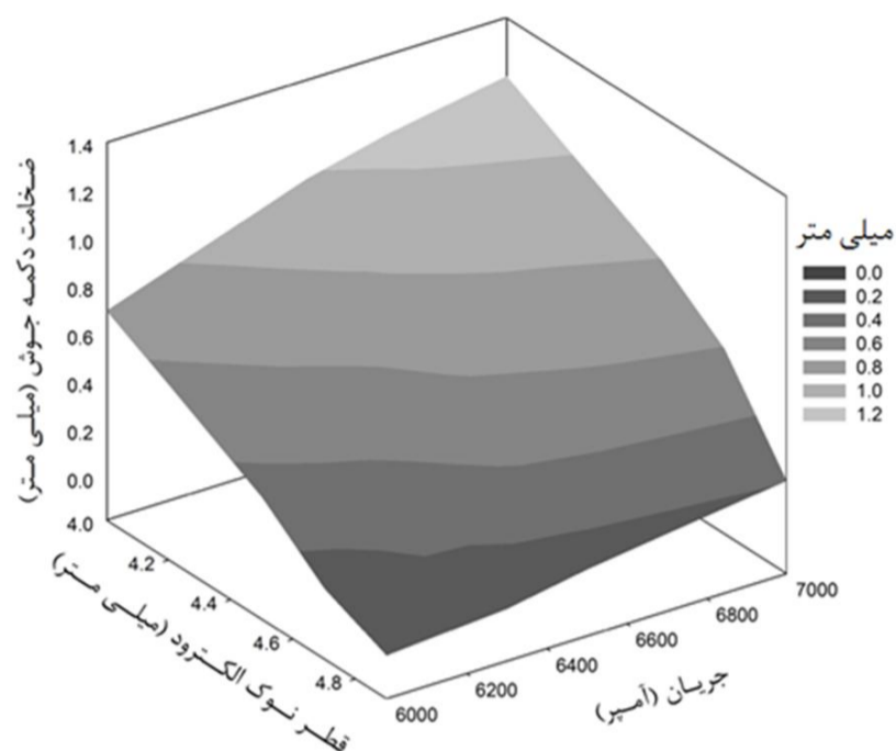
شکل 9 تأثیر متقابل جریان جوشکاری و قطر نوک الکتروود بر ضخامت دکمه جوش
