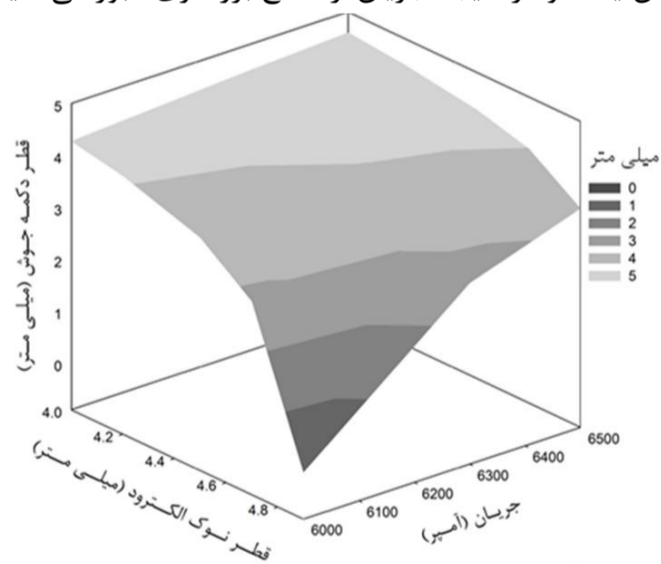
شکل 7 تأثیر همزمان جریان جوشکاری و قطر نوک الکتروود بر قطر دکمه جوش
