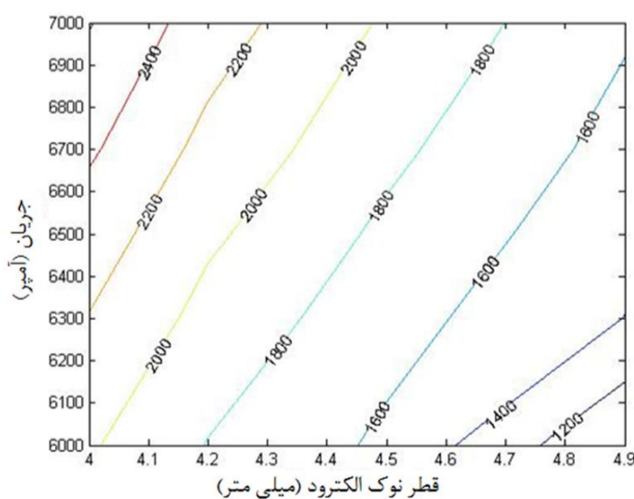
شکل 8 تأثیر متقابل جریان جوشکاری و قطر نوک الکتروود بر حداکثر دمایی دکمه جوش بر حسب درجه سانتی‌گراد
