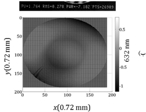
شکل 7 (الف) فرانس‌های سطح اولیه (ب) ماتریس اولیه سطح (با بزرگ‌نمایی \frac{1}{0.72} )
