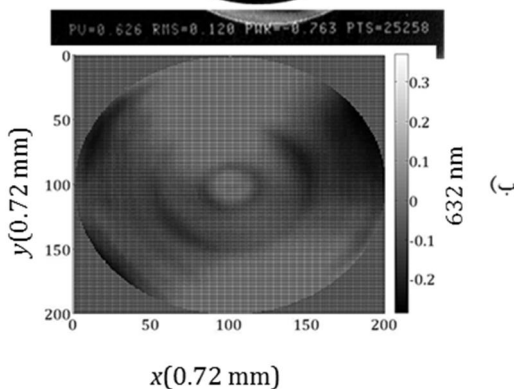
شکل 11 (الف) فرانس‌های سطح بعد از پرداخت (ب) ماتریس سطح بعد از پرداخت (با بزرگ‌نمایی \frac{1}{0.72} )
