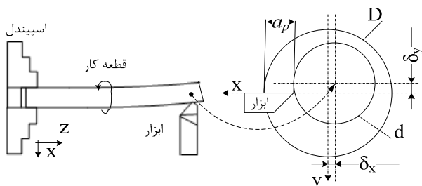
شکل ۵ برگشت فزنی قطعه کار در فرایند تراشکاری
