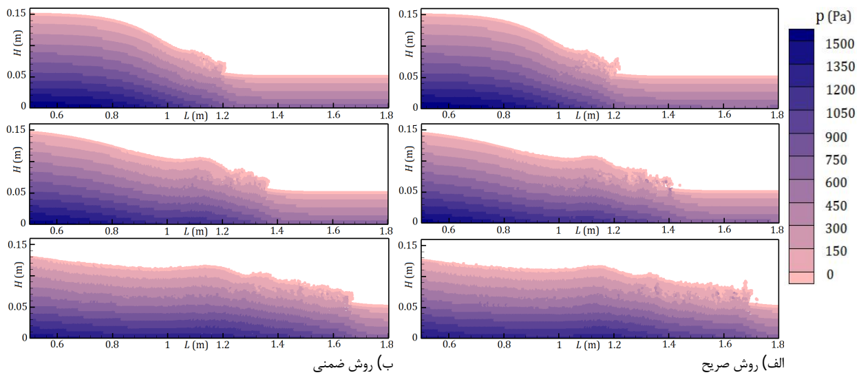
شکل 13 نتایج توزیع فشار روش های صریح و ضمنی پیشنهادی در زمان های 0.05، 0.75 و 1 ثانیه (از بالا به پایین)
