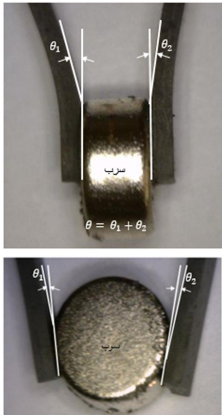
شکل 3 تصویر میکروسکوپی زاویه انحناء فک ناشی از خم شدن هر کدام از تیرها در اثر فشار بر جسم
