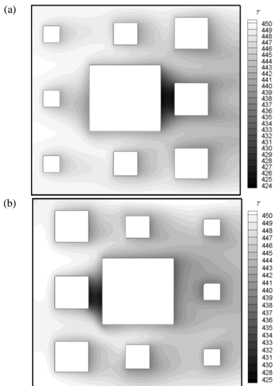
Fig. 18 Temperature (K) contour with specific area 0.56\text{m}^{-1} in a- small to large and b- large to small arrangements. شکل 18 نمایی از کانتهای دمایی (K) در محیط متخلخل با سطح مخصوص 0.56\text{m}^{-1} الف- کوچک به بزرگ و ب- بزرگ به کوچک
