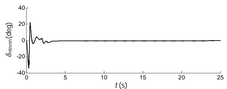
شکل 4 تغییرات سطوح کنترلی عرضی-سمتی
