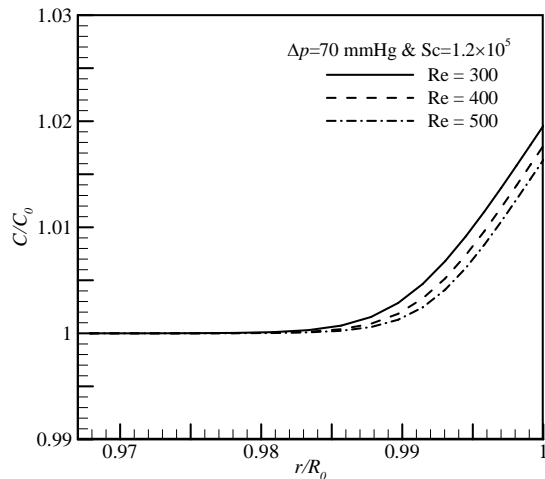
شکل 14 توزیع شعاعی ذرات لیپوپروتئین در ناحیه لومن در اعداد رینولدز مختلف
