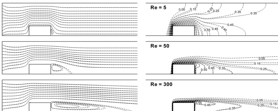
شکل ۴ میدان جریان (سمت چپ) و خطوط هم‌دما (سمت راست) برای نانو سیال آب+مس با \phi = 0.05 و (---) و آب خالص (—) در اعداد رینولدز مختلف و k^* = \infty و B = 5.33 ، Ri = 10
