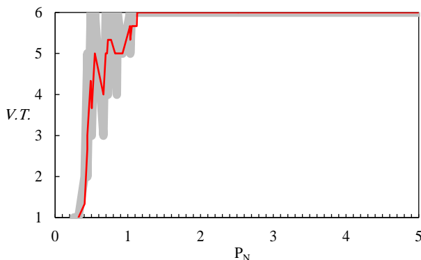
Fig. 8 Variation of V.T. vs. P_N شکل 8 تغییرات مرتبه گرداب (V.T.) نسبت به P_N
