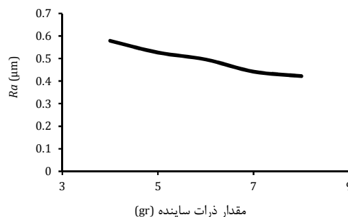
شکل ۱۴ میزان تغییر صافی سطح با تغییر مقدار ذرات ساینده
