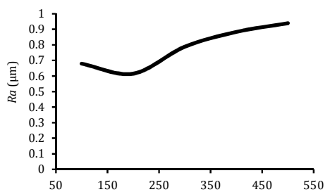
شکل ۹ تاثیر اندازه ذرات ساینده بر صافی سطح
