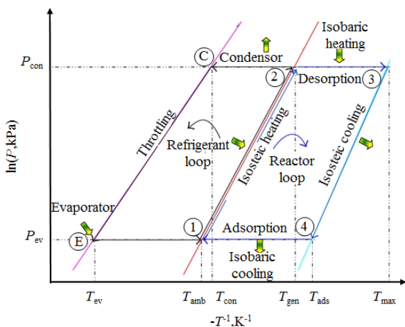
Fig. 3 Clapeyron diagram of adsorption refrigeration cycle [10] شکل 3 دیاگرام کلاپیرون چرخه تبرید جذبی [10]
