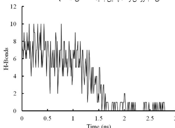
Fig.8 Changes in the number of hydrogen bonds during simulation شکل 8 تغییر تعداد پیوندهای هیدروژنی طی فرایند کشش مولکول
