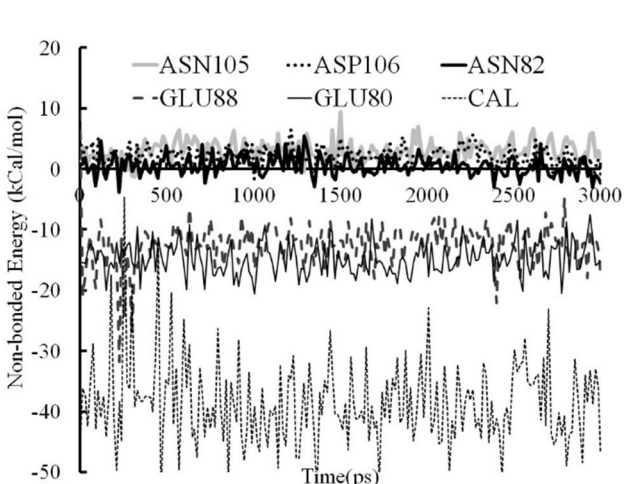
Fig. 10 The variation of non-bonded energies between FUC and CAL ion and its nearby residues during equilibration شکل 10 تغییرات انرژی ناپیوندی بین باقیمانده FUC با یون CAL و باقیمانده های مجاور این یون در طول به تعادل رسانی
