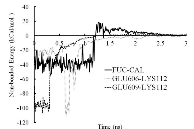
Fig. 11 The variation of non-bonded energies of the most effective residues in dissociation durrng pulling with constant velocity شکل 11 تغییرات انرژی ناپیوندی بین باقیمانده های مرزی که بیشترین تأثیر را در جدایش ایفا می کنند در طی کشیدن ساختار تحت کشش با سرعت ثابت
