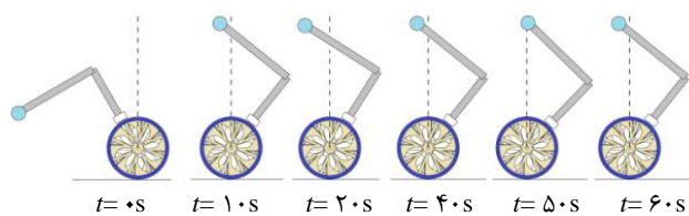
شکل ۲۴ تصویر ربات در طول زمان و اصلاح حالت خود جهت حفظ تعادل حین انجام فعالیت
