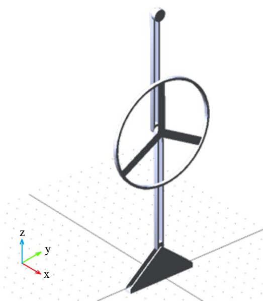
شکل ۴ مدل شبیه‌سازی شده از پاندول معکوس دوگانه با چرخ عکس‌العملی در نرم‌افزار آدامز
