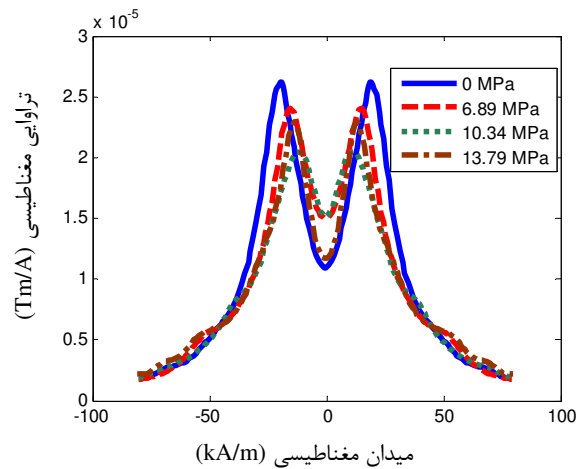
شکل ۷ نمودار تراوایی مغناطیسی ترفنل-دی برحسب میدان مغناطیسی در پیش بارهای مکانیکی مختلف
