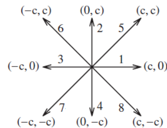
شکل ۲ مؤلفه سرعت گسسته \vec{e}_i برای مدل D_2Q_9
