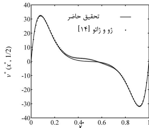
ب- نمودار مؤلفه عمودی سرعت بی بعد
