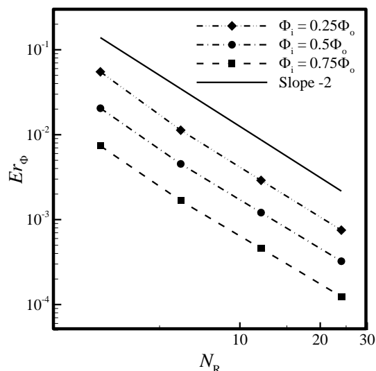
شکل ۹ تغییرات شاخص خطا نسبت به ابعاد شبکه
