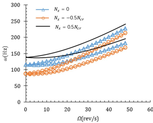
Fig. 16 The effect of axial load on frequency for n=4 شکل 16 اثر نیروی محوری روی فرکانس طبیعی برای n=4
