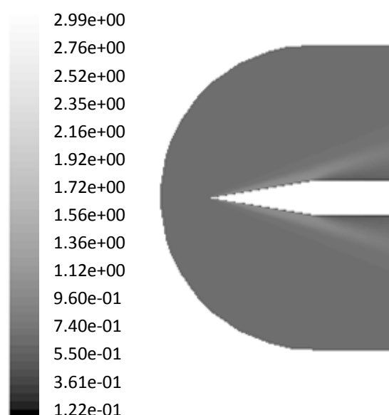
شکل ۹ کانتر دانسیته در صفحه تقارن پرتابه بعد از دائمی شدن جریان
