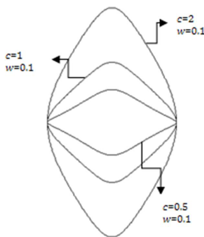
شکل 2 تأثیر پارامتر C بر هندسه گشودگی
