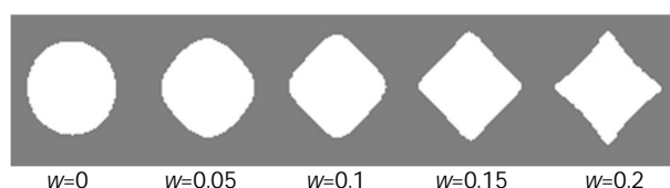
شکل 3 تأثیر پارامتر W بر هندسه گشودگی برای c=1
