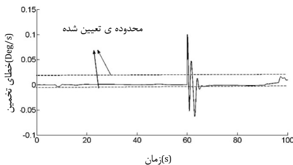
شکل ۸ شناسایی خرابی تمایل با استفاده از سنسور پیشنهادی
