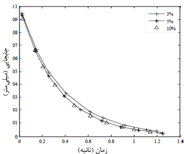
شکل ۲ پاسخ زمانی تیر هیبرید با ورودی ضربه
