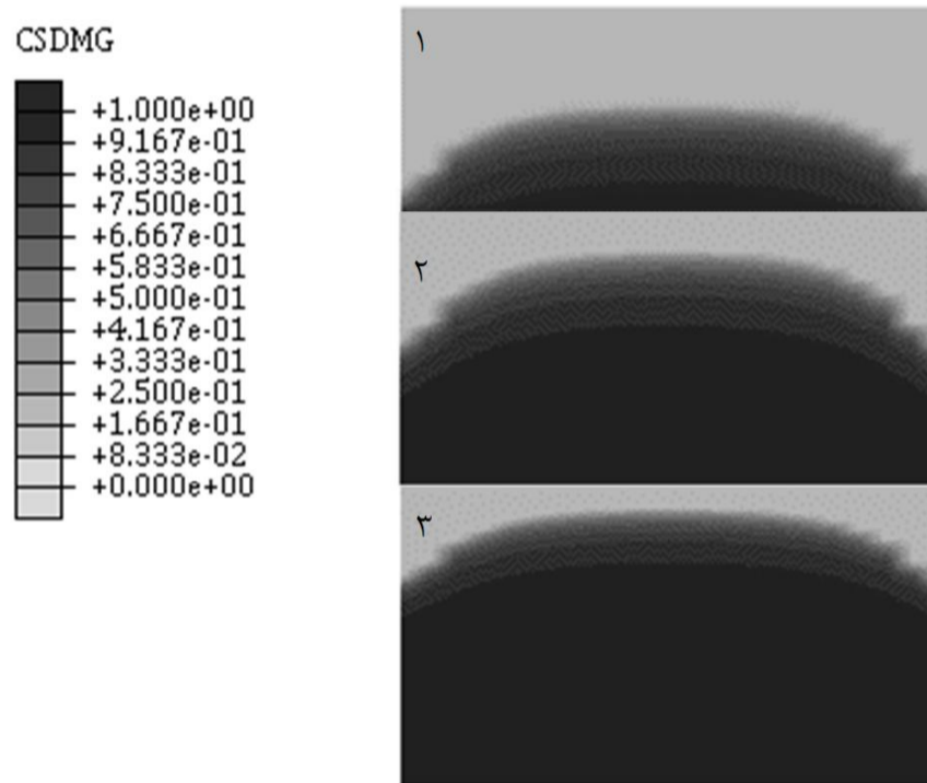
شکل ۲۴ پارامتر خرابی و جبهه ترک بدست آمده از مدل سازی عددی برای مود یک جدول ۵ چقرمگی شکست بین لایه ای مود دو (واحد N/m)
