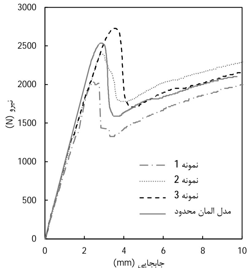
شکل 30 نمودار نیرو برحسب جابجایی تجربی و حاصل از مدل‌سازی عددی
