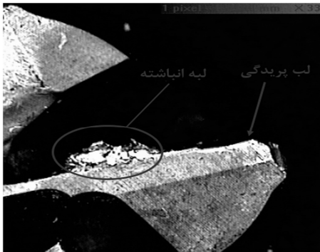
شکل ۳ تصویر لبه ابزار استفاده‌شده در فرزکاری ماریچج
