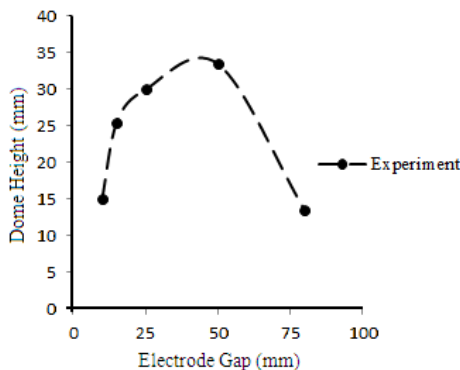
Fig. 17 The effect of electrode gap on dome height شکل 17 اثر فاصله بین الکتروودها بر روی ارتفاع گنبد
