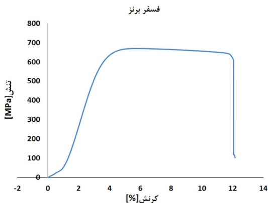
شکل 2 منحنی تنش - کرنش فسفر برنز
