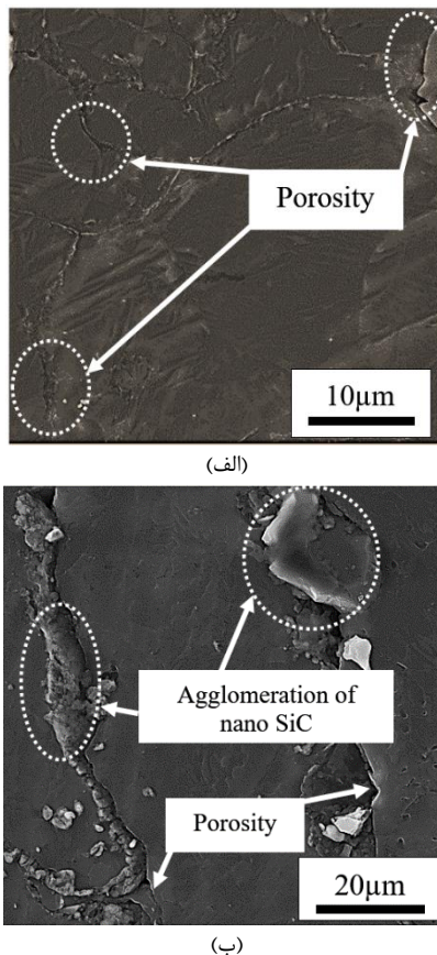
Fig. 7 SEM micrographs of compacted specimen: a- Mg-0vol% SiC, b- Mg-3vol% SiC شکل 7 تصاویر میکروسکوپ الکترونی نانو کامپوزیت Mg-SiC: الف- Mg-0vol% SiC، ب- Mg-3vol% SiC
