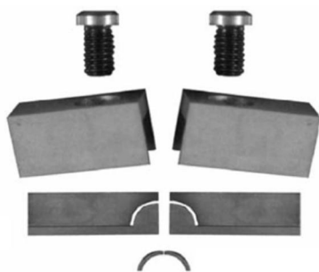
شکل 16 فیکسچر و نمونه آزمایش خمشی سه نقطه [29]
