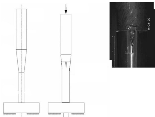
شکل 17 روش آزمایش قالب مخروطی داخلی [28]
