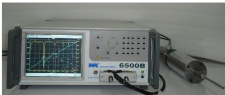
شکل 2 اندازه‌گیری فرکانس رزونانس ترانسدیوسر
