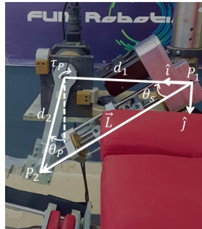
Fig. 9 Parameters used in mathematical modeling of FUM-Physio robot شکل 9 پارامترهای مورد استفاده در مدل‌سازی ریاضی ربات فام-فیزیو
