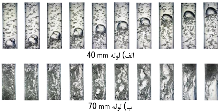
شکل 16 الگوی جریان در فریم‌های متوالی برای دو لوله به قطر داخلی 40 mm و 70 mm در ارتفاع 3/22 m برای j_G=0/379 m/s و j_L=0/368 m/s
