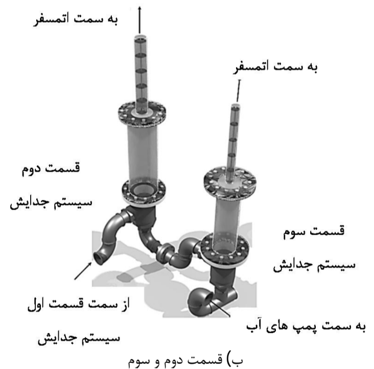
شکل 3 نمایی از سیستم جدایش سیستم آزمایشگاهی
