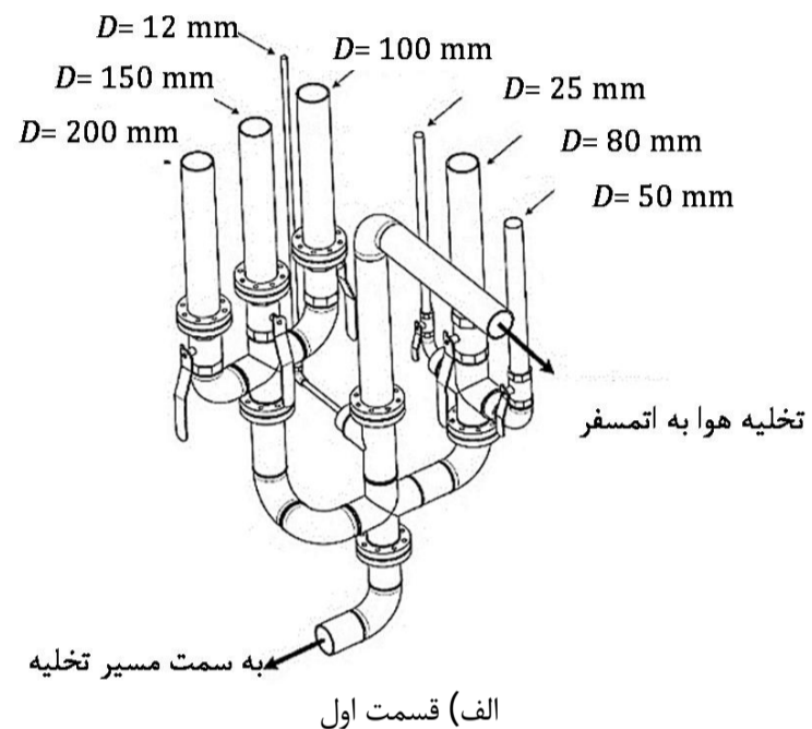
شکل 2 طرح‌واره محفظه اختلاط طراحی شده
