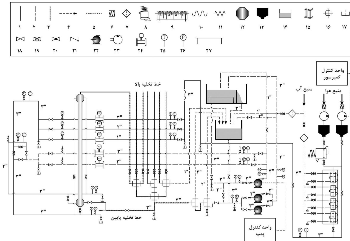
شکل 1 نقشه سیستم آزمایشگاهی عمودی: (1) خط هوا، (2) خط آب، (3) خط تخلیه، (4) خط فرار هوا/ونت، (5) خط الکتریکی، (6) فیلتر هوا، (7) فیلتر آب، (8) تنظیم کننده فشار، (9) سیستم سرمایش هوا، (10) لوله قابل انعطاف، (11) ضربه گیر، (12) مخزن اختلاط، (13) تانک هوا، (14) تانک آب، (15) لوله آزمایش، (16) چهار راه، (17) تخلیه (درین)، (18) شیر فلکه‌ای، (19) شیر سماوری، (20) شیر فلکه‌ای (هوا)، (21) شیر یک طرفه، (22) پمپ آب، (23) کمپرسور هوا، (24) فلومتر هوا/آب، (25) دماسنج، (26) فشارسنج، (27) حباب‌گیر
