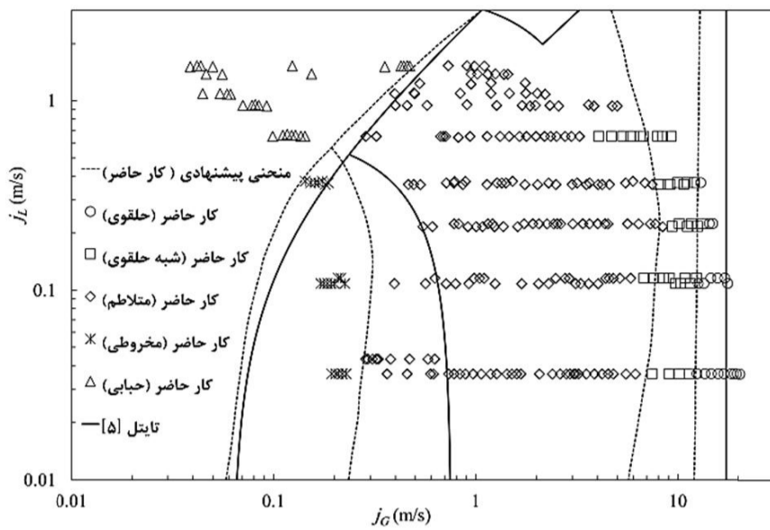
شکل 14 نقشه الگوی جریان برای لوله به قطر داخلی 70 mm در L/D=46
