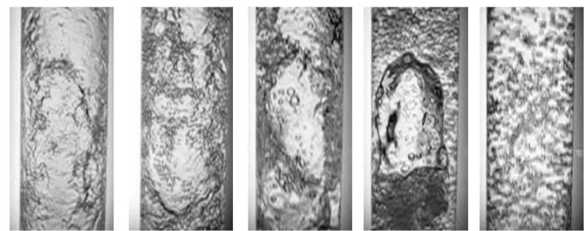
شکل 12 الگوهای جریان در لوله عمودی به قطر داخلی 70 mm (الف) حبابی (ب) اسلاگ (ج) متلاطم (د) شبه-حلقوی (ه) حلقوی
