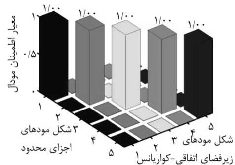
شکل ۷ مقایسه شکل مودهای محاسبه شده به روش زیر فضاهای اتفاقی بر مبنای کواریانس و روش اجزای محدود-شاخص پیشنهادی
