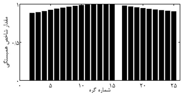
شکل ۴ مقدار شاخص همبستگی برای درجات آزادی جابه‌جایی
