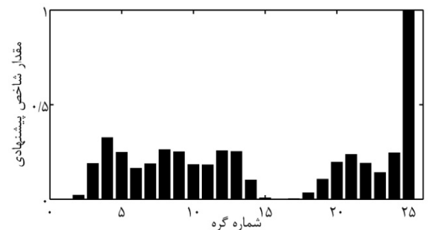
شکل ۳ مقدار شاخص پیشنهادی برای درجات آزادی جابه‌جایی
