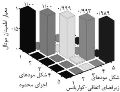
الف) معیار اطمینان مودال با اضافه شدن ۵٪ نویز-شاخص پیشنهادی
