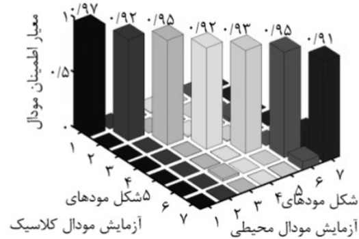
شکل ۲۳ مقایسه شکل مودالهای حاصل از آزمایش‌های مودال کلاسیک و مودال محیطی به کمک معیار اطمینان مودال
